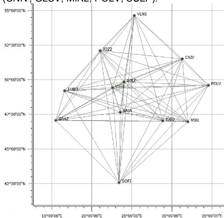
Рис. 1. Мережа опорних GNSS станцій (GIPSY)
