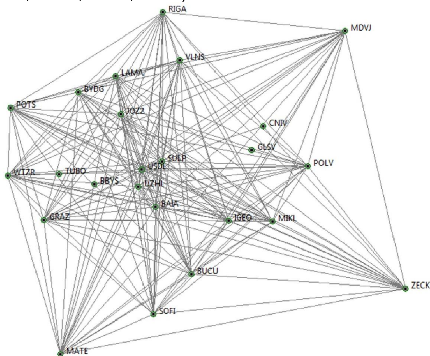
Рис. 2. Мережа опорних GNSS станцій (GAMIT)
